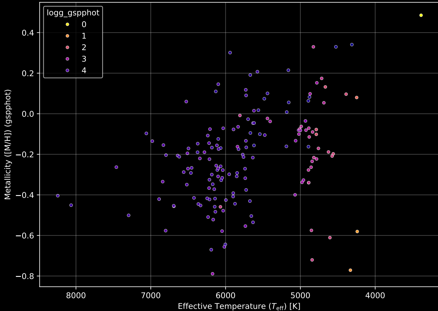
GALAH DR4 Field: [7128] Stellar Population Parameters (n= 161)
